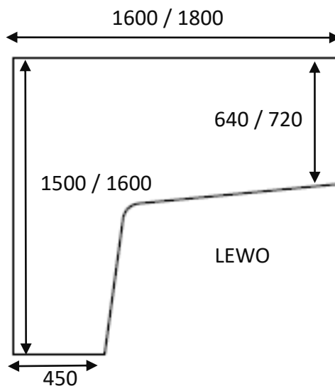
Blaty formy kompaktowe
