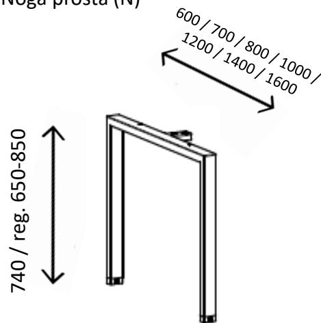
Noga prosta (N)
