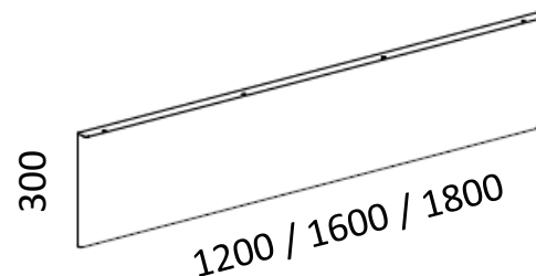
Pionowy kanał kablowy magnetyczny
