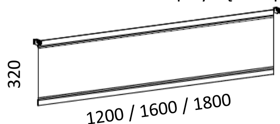
Osłona z siatki mesh przykręcana pod blatem
